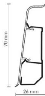
LISTWA PCV - Arbiton Indo h=7 cm
